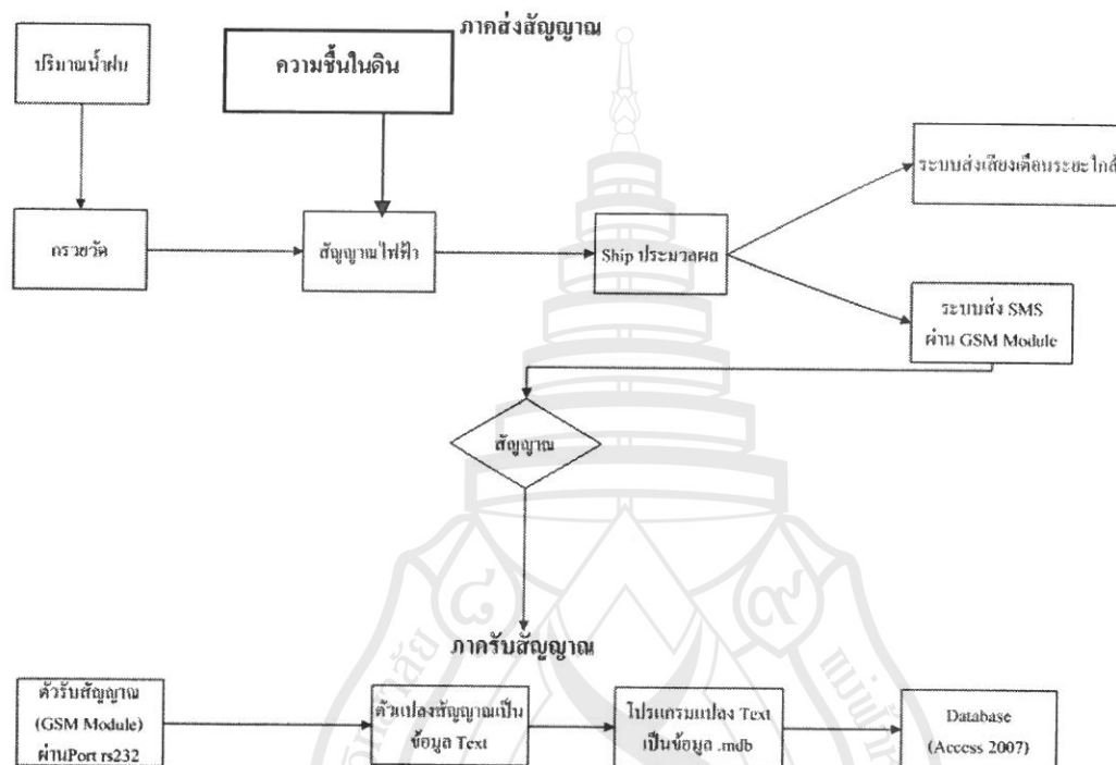
ภาพที่ 2 แผนภาพ (Flow Chart) ระบบวัดปริมาณน้ำฝน ปริมาณน้ำในดิน
