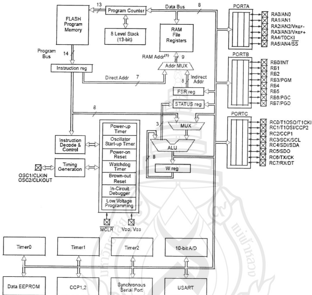
ภาพที่ 3-13 ผังโคอะแกรมของ PIC 16F877
