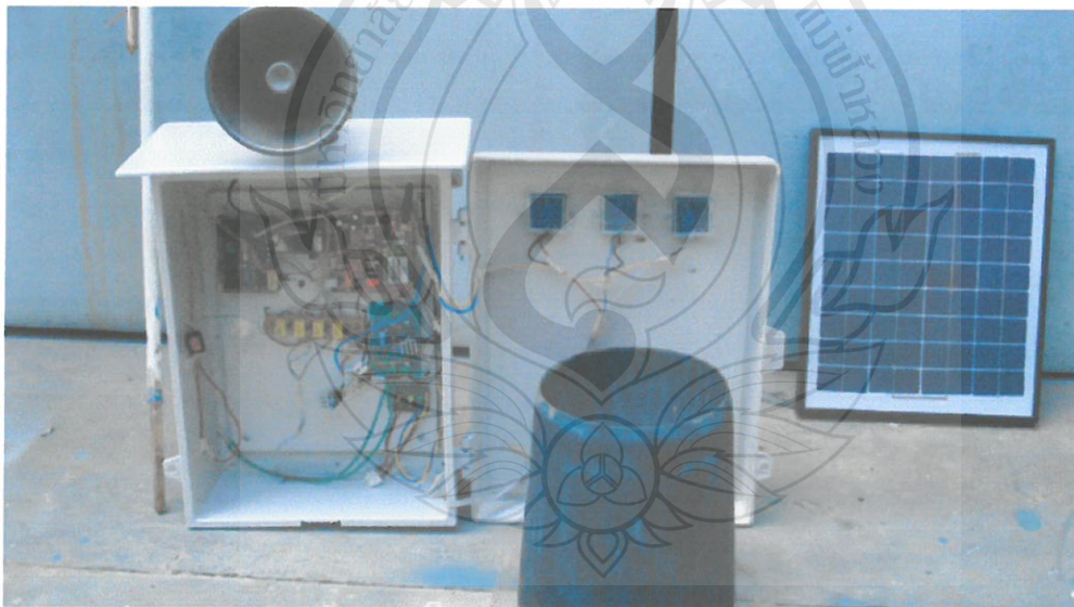
ภาพที่ 4-30 รูปแสดงอุปกรณ์ที่พร้อมติดตั้ง
