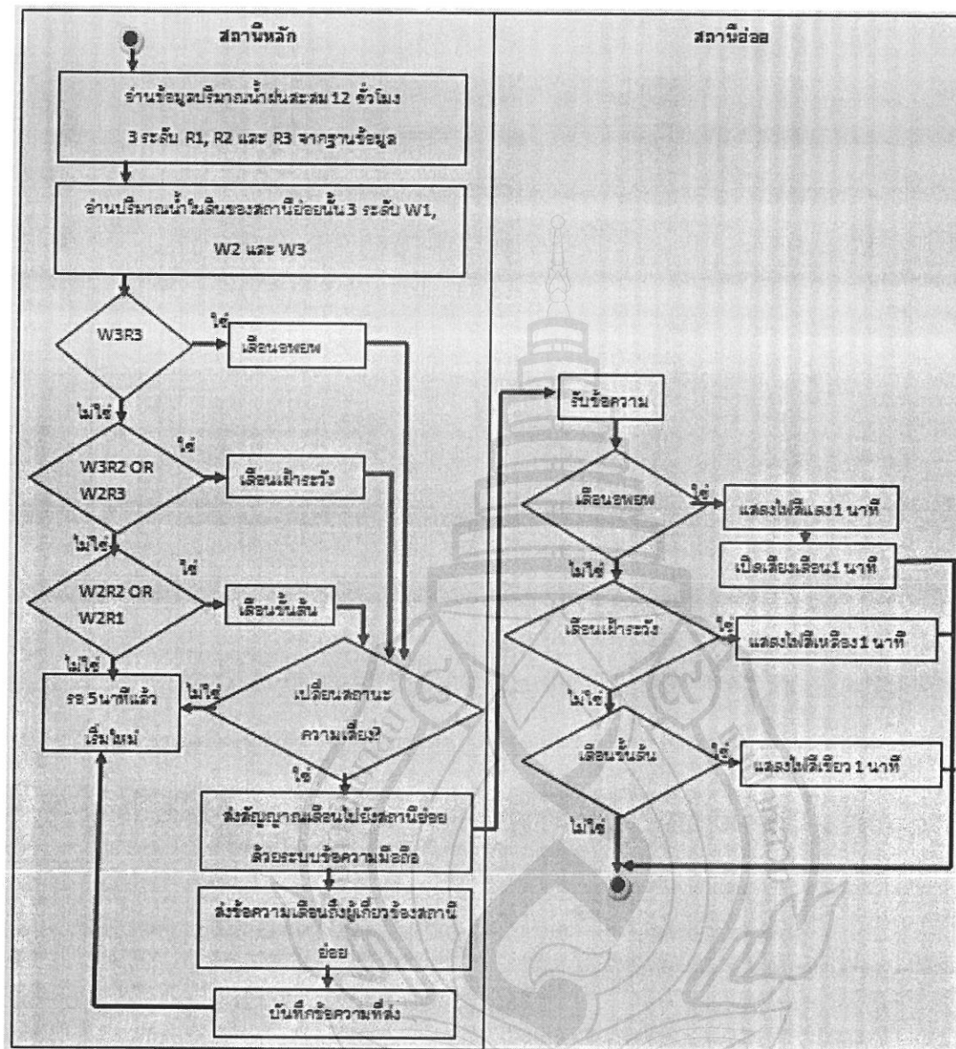
ภาพที่ 5 แผนภาพ (Flow Chart) การทำงานของระบบ
