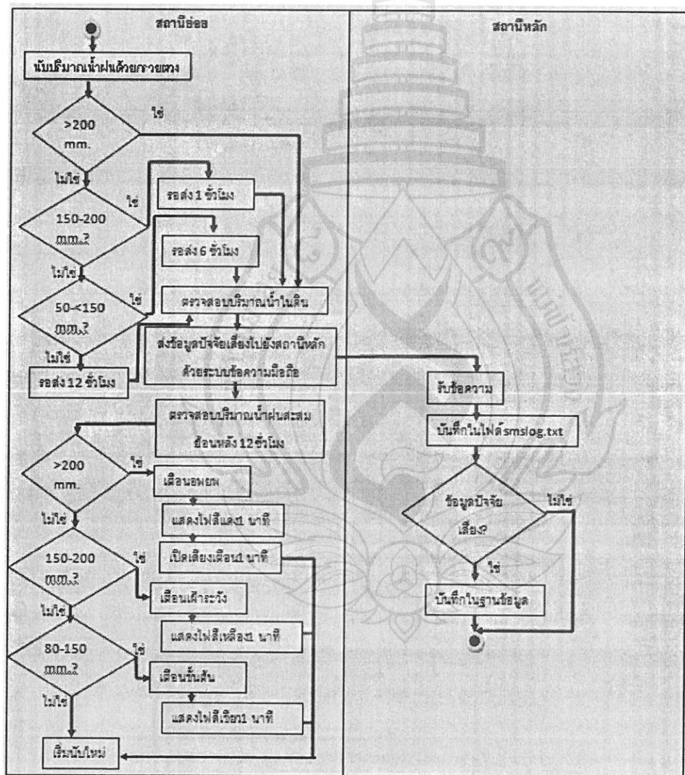
ภาพที่ 4 แผนภาพ (Flow Chart) แผนผังการทำงานของระบบในการเก็บและบันทึกค่าปัจจัยเสี่ยง
