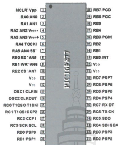
ภาพที่ 3-12 การจักระบบของ PIC16F877
