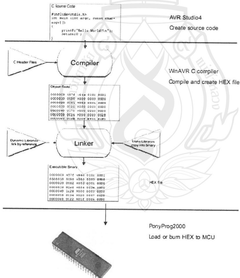
ภาพที่ 3-8 แปลนขั้นตอนการเขียนโปรแกรมลงในไมโครคอนโทรลเลอร์
