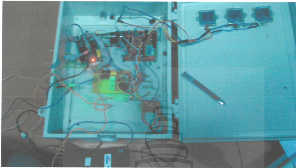
ภาพที่ 4-29 แสดงการเชื่อมต่อของภาคส่ง
