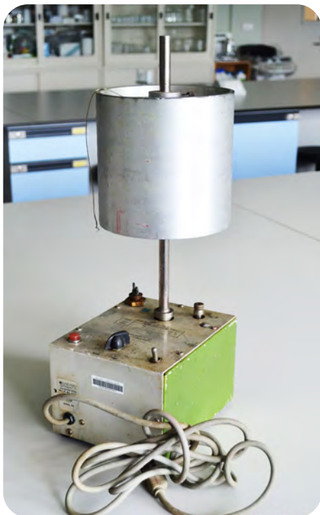
เครื่อง Kymograph ที่ได้รับมาจากภาควิชาสรีรวิทยา คณะแพทยศาสตร์ศิริราชพยาบาล
