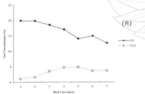
รูปที่ 4- 8 การเปลี่ยนแปลงปริมาณก๊าซภายในภาชนะบรรจุของสับปะรดตัดแต่งพร้อมบริโภคที่บรรจุด้วยฟิล์ม PVC ขนาดความหนา 8 ไมครอน (ก) PVC ขนาดความหนา 12 ไมครอน (ข) ถุง PP (ค) ถุง PE (ง) ณ อุณหภูมิ 15 องศาเซลเซียส
