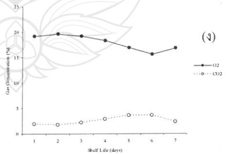
รูปที่ 4- 8 การเปลี่ยนแปลงปริมาณก๊าซภายในภาชนะบรรจุของสับปะรดตัดแต่งพร้อมบริโภคที่บรรจุด้วยฟิล์ม PVC ขนาดความหนา 8 ไมครอน (ก) PVC ขนาดความหนา 12 ไมครอน (ข) ถุง PP (ค) ถุง PE (ง) ณ อุณหภูมิ 15 องศาเซลเซียส
