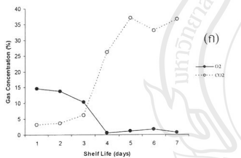
รูปที่ 4- 7 การเปลี่ยนแปลงปริมาณก๊าซภายในภาชนะบรรจุของสับปะรดตัดแต่งพร้อมบริโภคที่บรรจุด้วยฟิล์ม PVC ขนาดความหนา 8 ไมครอน (ก) PVC ขนาดความหนา 12 ไมครอน (ข) ถุง PP (ค) ถุง PE (ง) ณ อุณหภูมิ 10 องศาเซลเซียส
